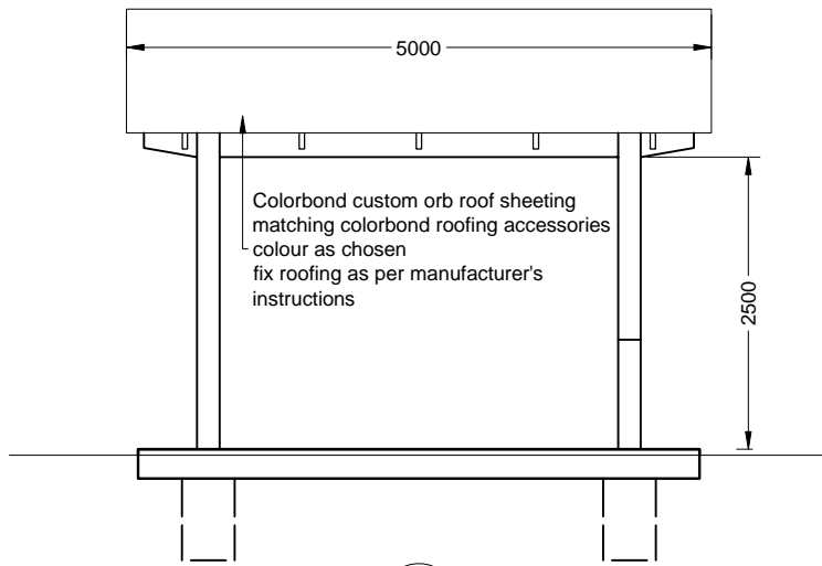
ELEVATION 1 LOW SIDE Scale: 1:50
