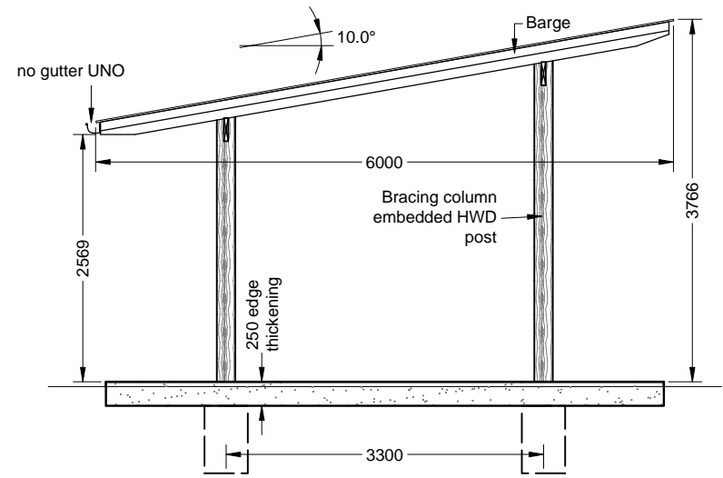
ELEVATION 2 END Scale: 1:50
