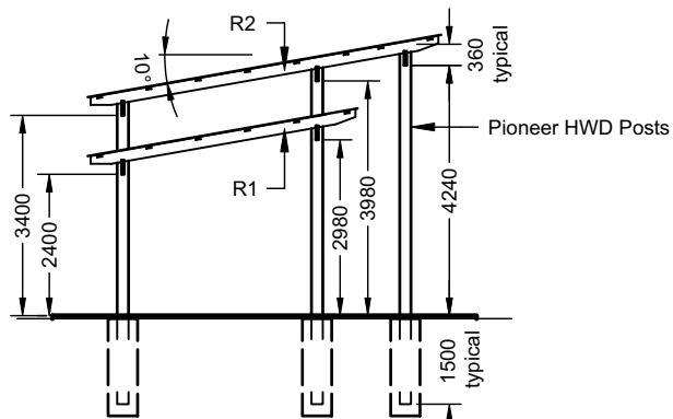
ELEVATION 2/1 SIDE Scale: 1:100
