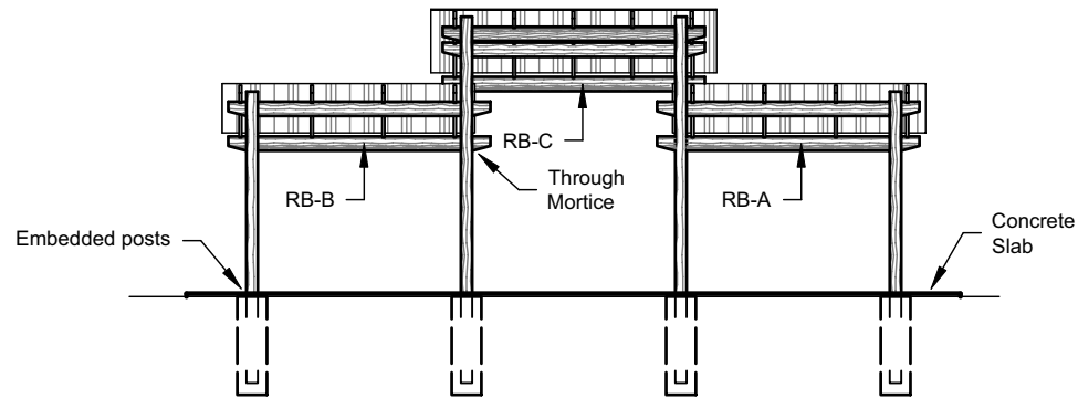
ELEVATION 1/1 FRONT Scale: 1:100
